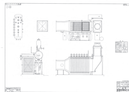
WBF-330型外形図
