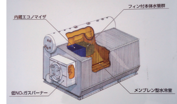
YSG-25型ボイラ構造
