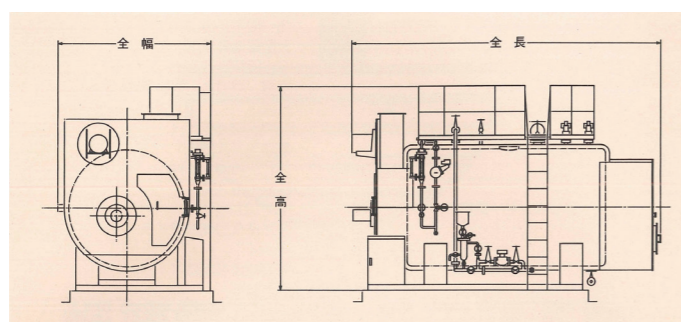
YM型ボイラー外形図
