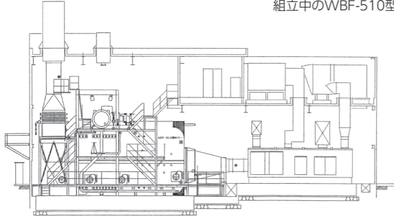
ガスタービンとWBF-510型排熱ボイラ
